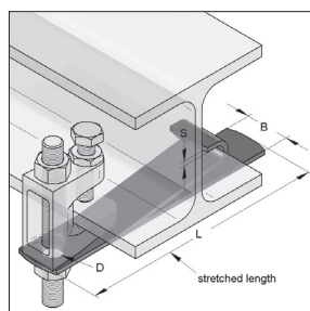
Pletina de seguridad
