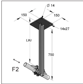
Consola para Punto Fijo 50/38/750
