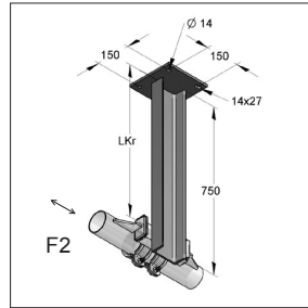
Consola para Punto Fijo 120/55/750
