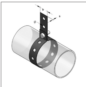
Montaje de cinta perforada de acero -PLASTAHL-
