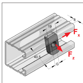
Tuerca carril
