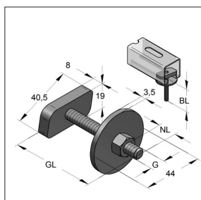
Tornillo cab. martillo
