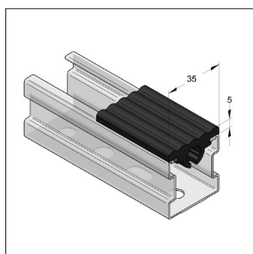
STEX 35 perfil de goma
