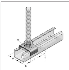
Grapa de fijación
