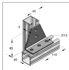
Placa de conexión T, c/ángulo 90°
