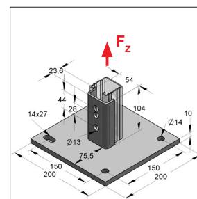
Soporte con placa cuadrada para carril-C
