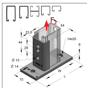
Soporte vertical para carril-C
