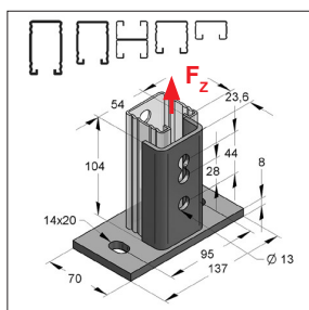
Soporte horizontal para carril-C
