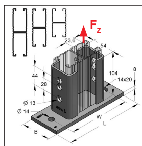
Soporte para carril doble-C
