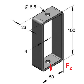
Soporte colgante 2-taladros 100/50/4
