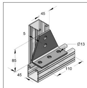
Placa de conexión T, c/ángulo 90°
