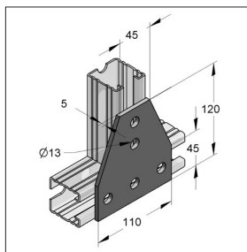
Placa de conexión T
