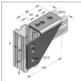
Conector angular izquierda, 4-taladros
