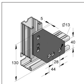
Placa de conexión angular, 4-taladros
