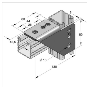
Conector angular derecha, 4-taladros
