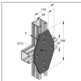
Placa de conexión en cruz
