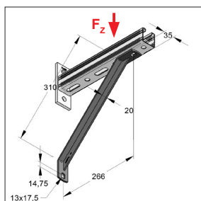
Apoyo / tirante 45° corto
