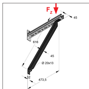
Apoyo / tirante 45° largo
