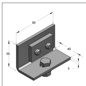
Ángulo adaptador
