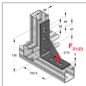
Ángulo reforzado 5-taladros 40/5
