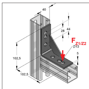
Ángulo reforzado 4-taladros 40/5
